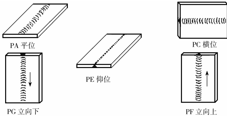
(a) 对接焊缝
