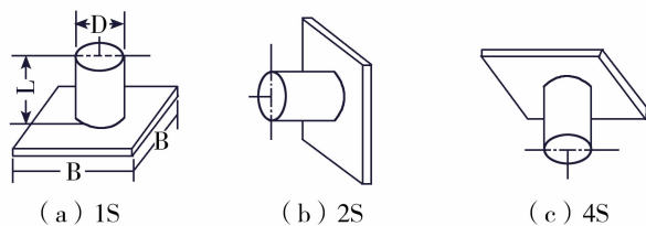
A 螺柱焊缝——试验位置
