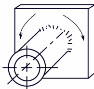
PG 管：固定 轴线：水平 焊接：向下立焊
