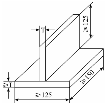
T 为试板厚度
