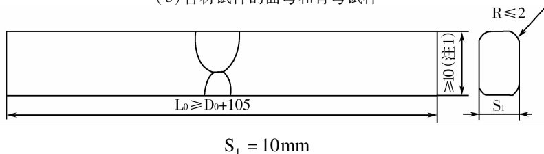
(c) 对接侧弯试样
