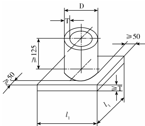
l_1 为试板长度 D 为管外径 T 为管壁厚
