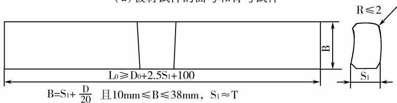
(b) 管材试件的面弯和背弯试样
