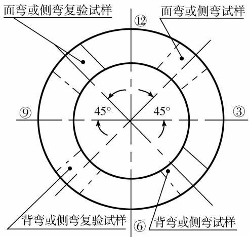
图 3(a) 管材试件弯曲试样的截取位置
