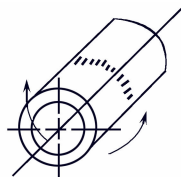
PF 管：固定 轴线：水平 焊接：向上立焊
