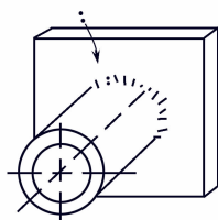
PB 管：转动 轴线：水平 焊接：平角焊
