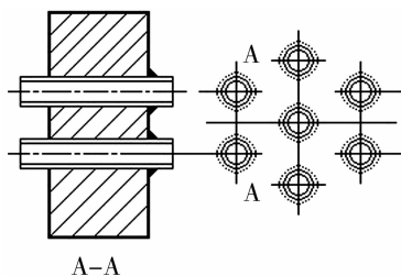
图 1 管子—管板示意图
