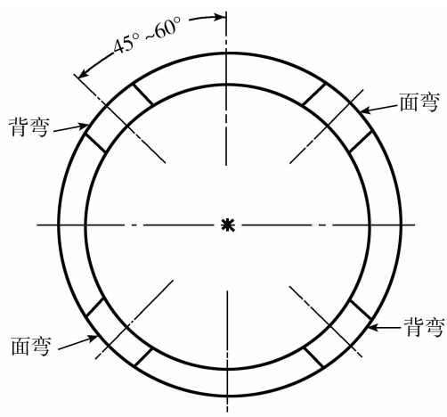
图 3(b) 表 1 注(3) 焊接位置弯曲试样的截取位置
