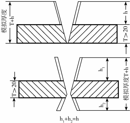
图 5 模拟厚板焊接试样
