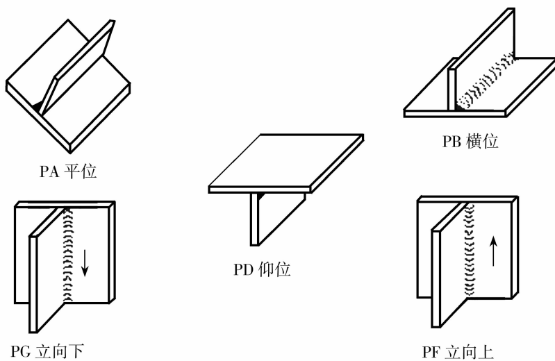
(b) 角焊缝
