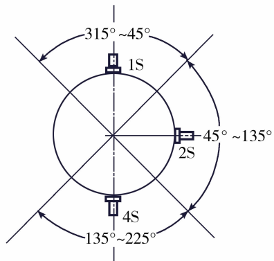
B 螺柱焊缝——焊接位置
