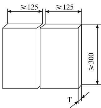
T 为试板厚度
