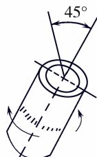
H-L045 管：固定 轴线：倾斜45度 焊接：向上立焊
