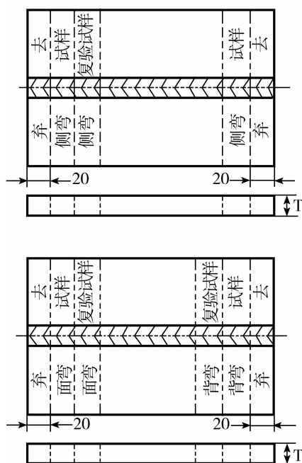
(a) 板材对接焊缝试件
