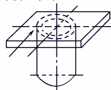
PD 管：固定 轴线：垂直 焊接：仰角焊
