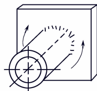
PF 管：固定 轴线：水平 焊接：向上立焊
