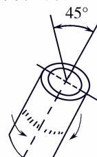
J-L045 管：固定 轴线：倾斜45度 焊接：向下立焊
