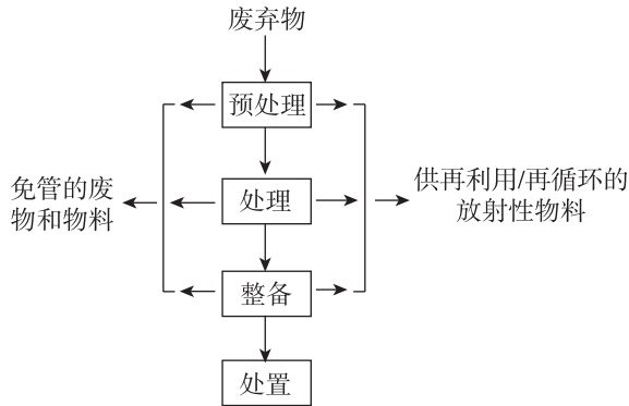
图1 放射性废物管理的基本步骤
